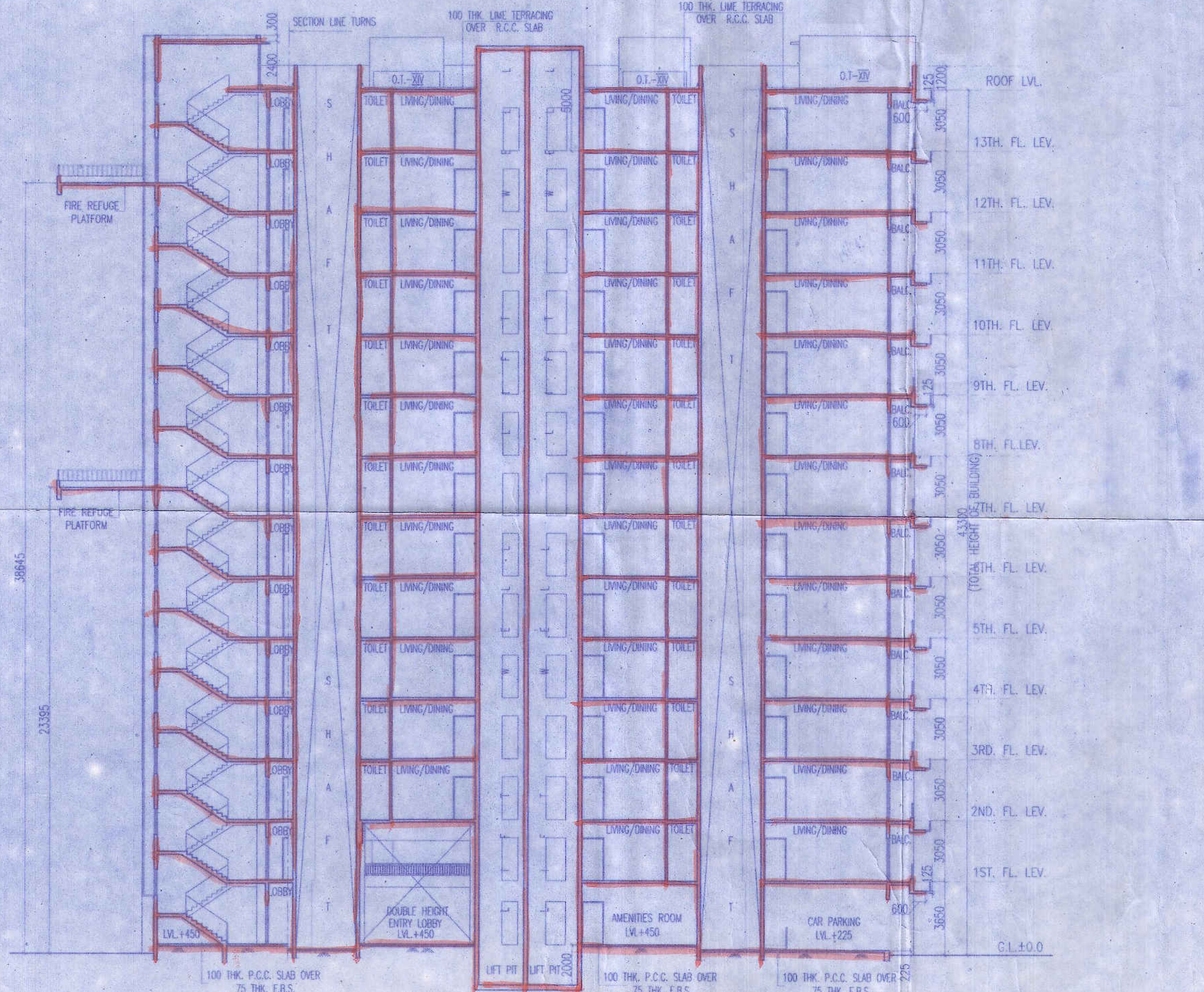
SECTION : U-U
